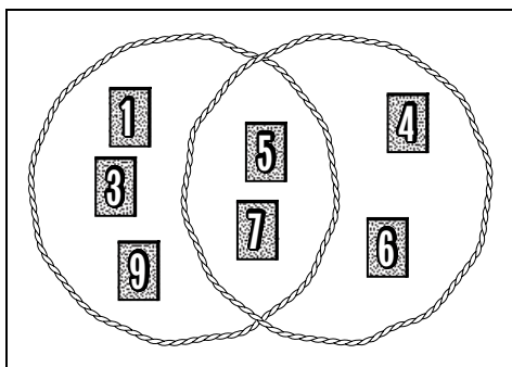
Рис. 47. Пересекающиеся множества.
